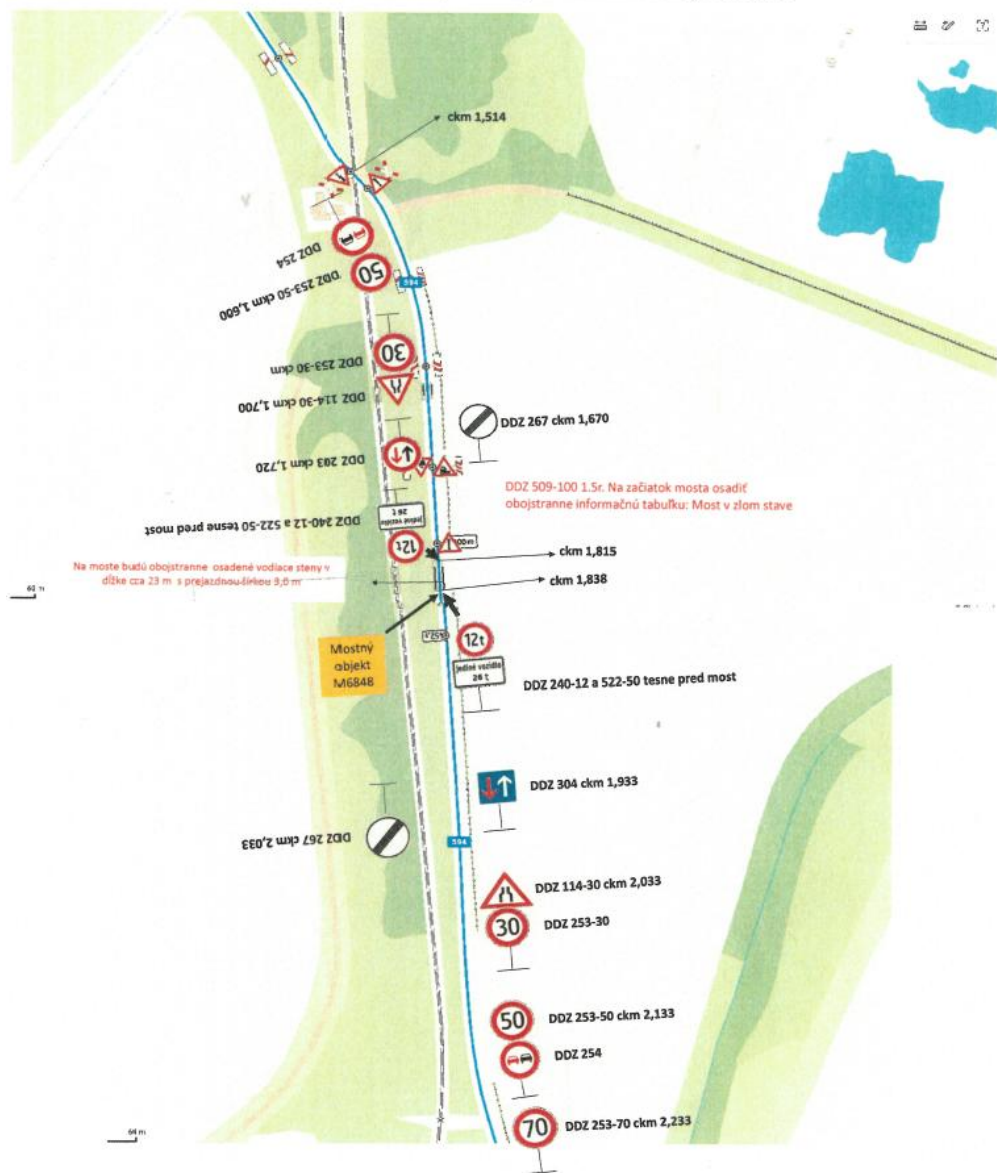
Návrh dočasného dopravného značenia na ceste II/594 na moste M6848 (ev.č. 594-005) Most cez inundačné územie pri obci Rapovce
