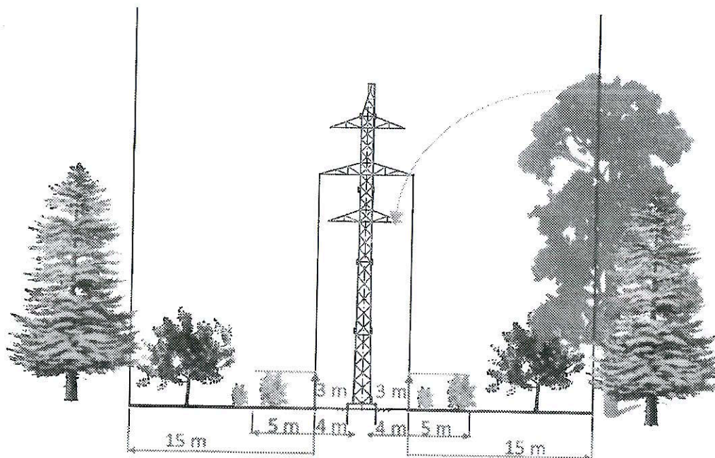
Obr. 2 Ochranné pásmo vonkajšieho nadzemného elektrického vedenia VVN. Červenou farbou je zvýraznený strom s potenciálne nebezpečnou vzdialenosťou dopadu.
