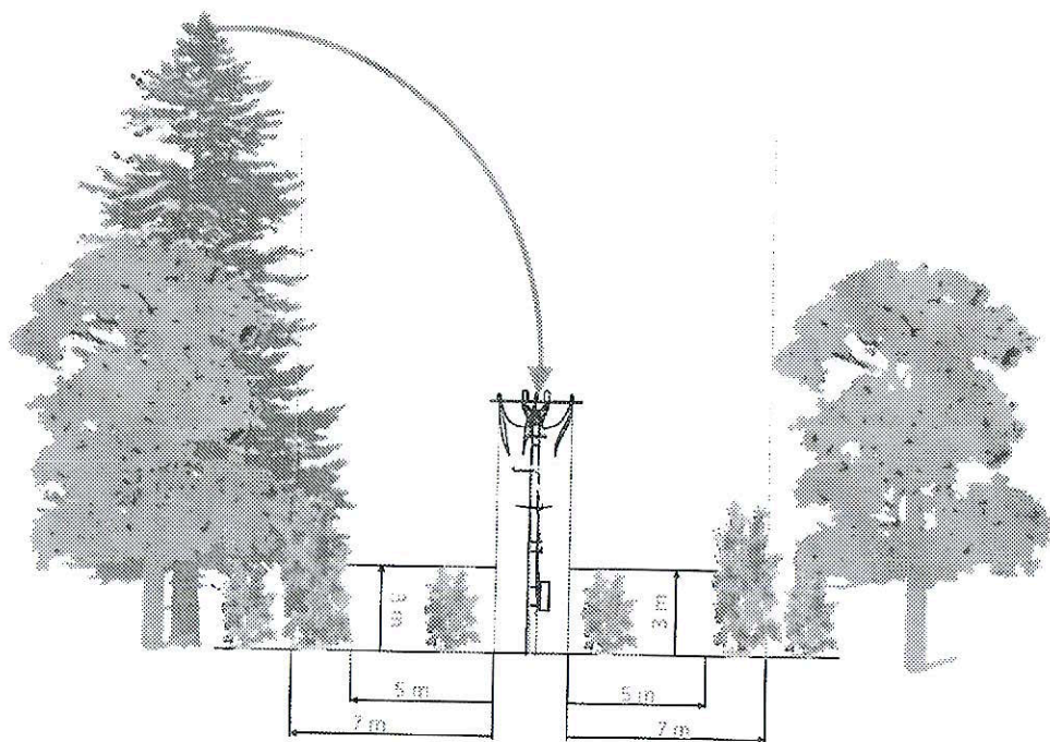
Obr. 1 Ochranné pásmo vonkajšieho nadzemného elektrického vedenia VN. Červenou farbou je zvýraznený strom s potenciálne nebezpečnou vzdialenosťou dopadu.
